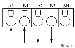
弹簧式总线连接器
