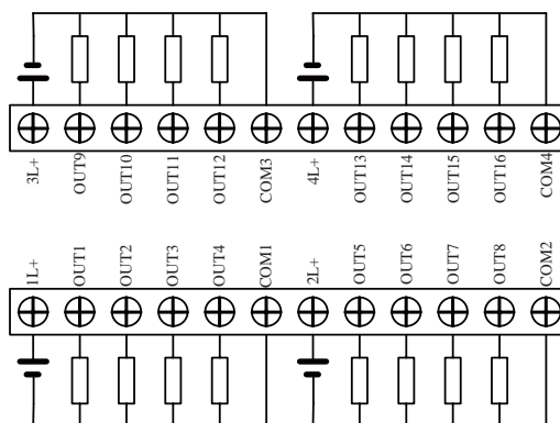
输出信号连接器
