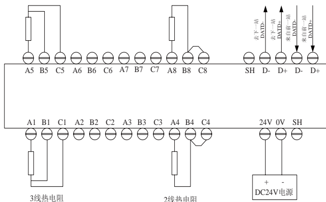
接线图
