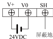
插拔式电源供电连接器
